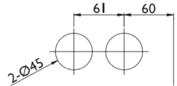
Bohrschema
