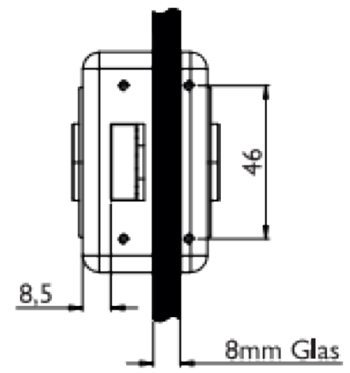
Bohrschema
