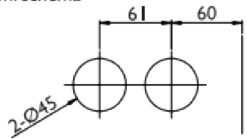
Bohrschema
