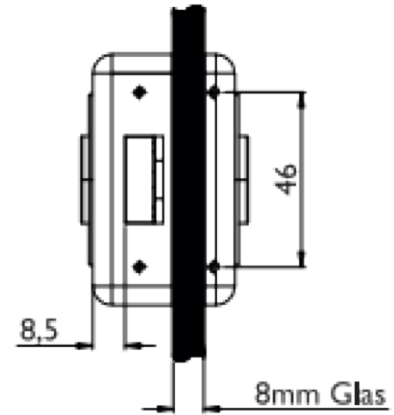
Bohrschema
