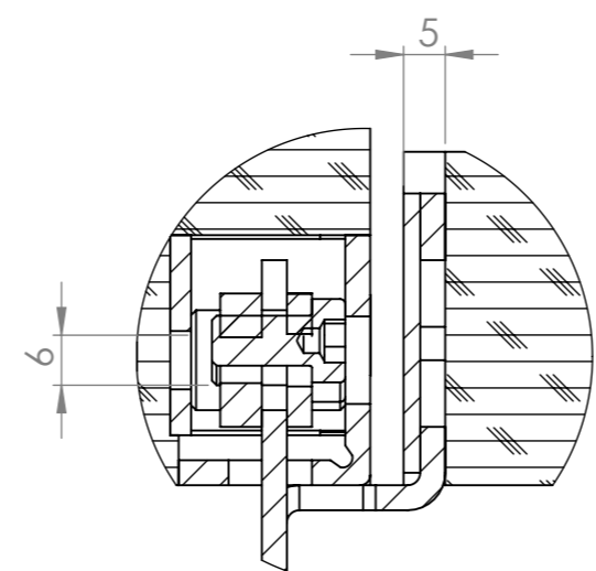
DETAIL C MAßSTAB 1 : 1
